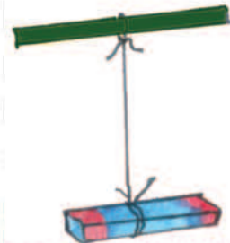
ଚିତ୍ର 13.7 ତୁମ୍ବକ ଦ୍ଵାରା ଦିଗ ନିର୍ଣ୍ଣୟ
