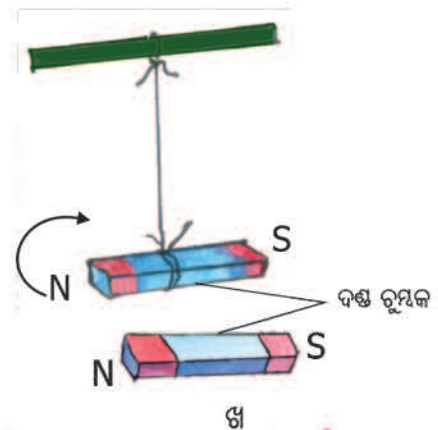
ଚିତ୍ର 13.10 ରୁମ୍ଭକୀୟ ବିକର୍ଷଣ
