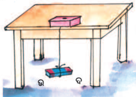
ଚିତ୍ର 13.8 ଦିଗ ଦର୍ଶାଉଥିବା ଦଣ୍ଡତୁମ୍ବକ
