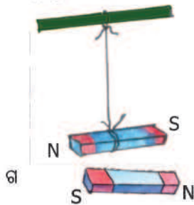
ଚିତ୍ର 13.11 ତୁମ୍ଭକାୟ ଆକର୍ଷଣ
