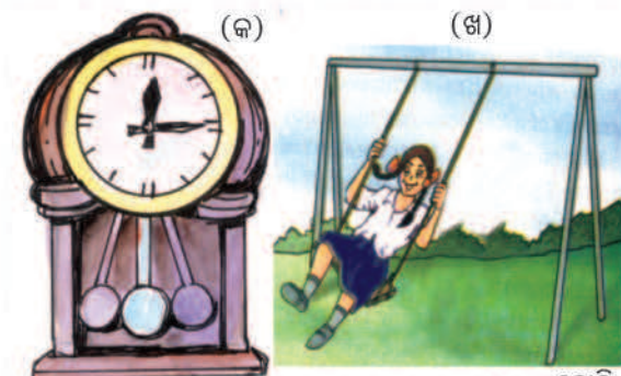
ଚିତ୍ର 11.5 ଦୋଳନ ଗତି
