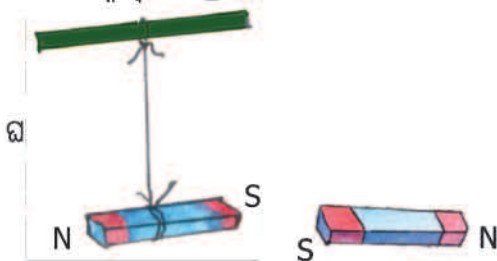
ଚିତ୍ର 13.12 ତୁମ୍ଭକାୟ ବିକର୍ଷଣ
