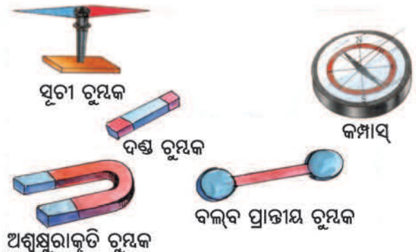
ଚିତ୍ର 13.3 ବିଭିନ୍ନ ଆକୃତିର ଚୁମ୍ବକ
